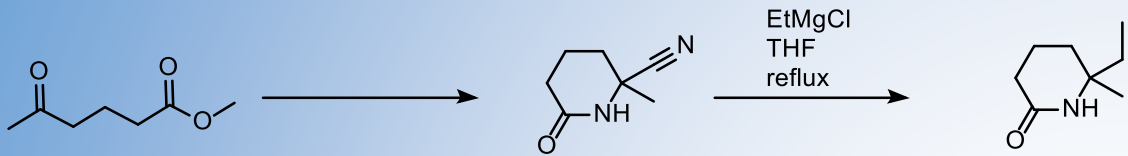
Реакція Бріллянта
