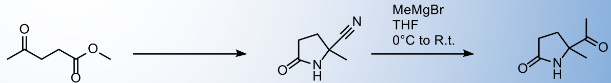
Реакція Грін'яра
